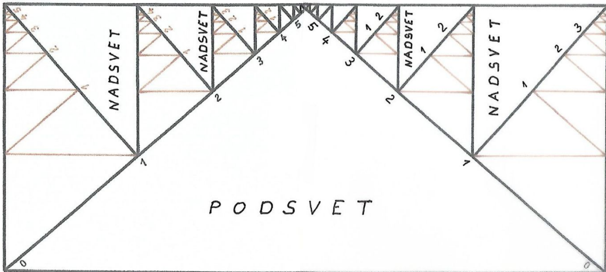
Slika 7: Struktura v globini duhovnega oceana.
