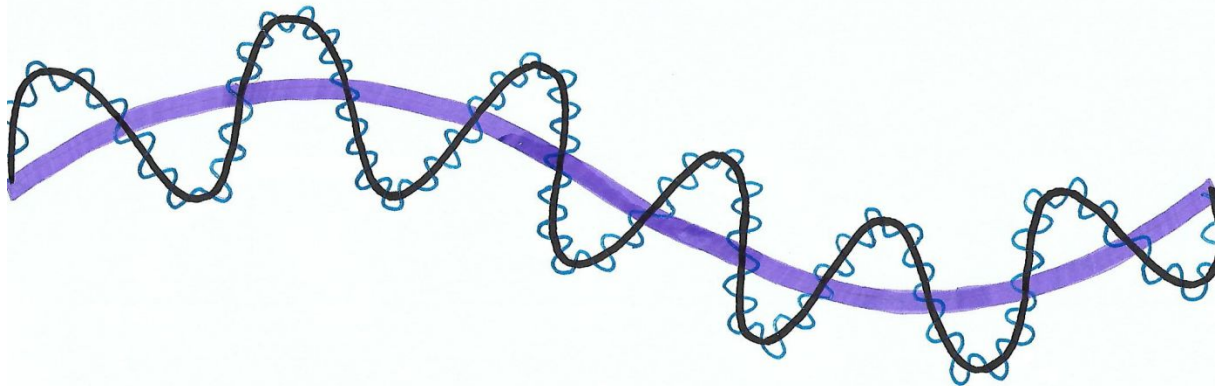
Slika 4: Osnovni val in višji harmoniki.
